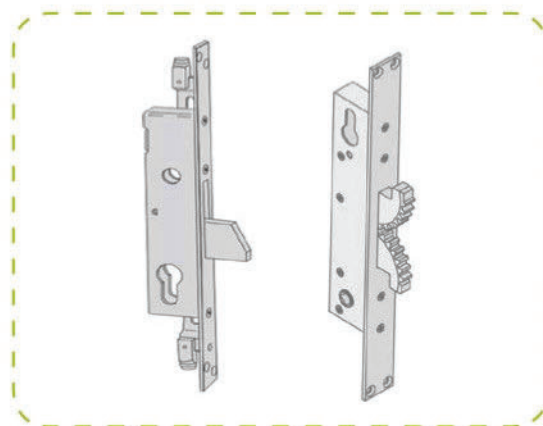
Dettaglio serratura cilindro europeo
