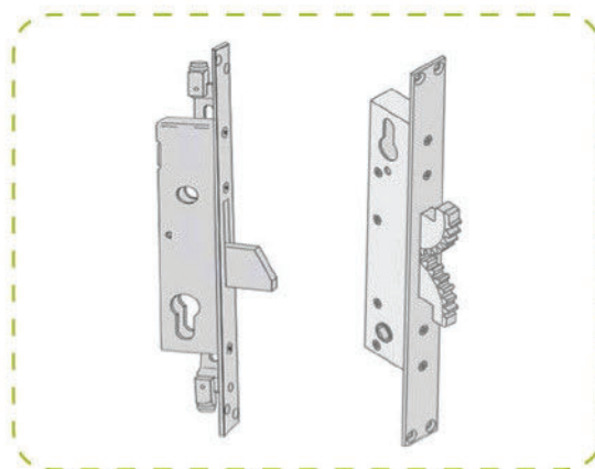
Standard Bunkerlocks Dettaglio serratura cilindro europeo
