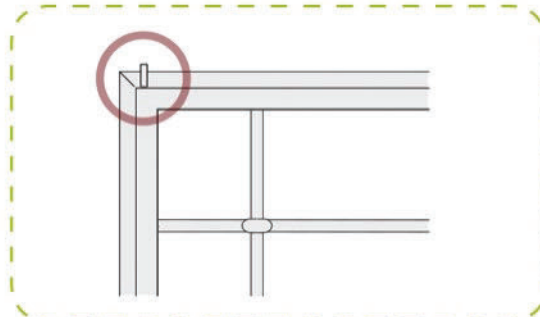
3. Anta con asta da 10 mm
