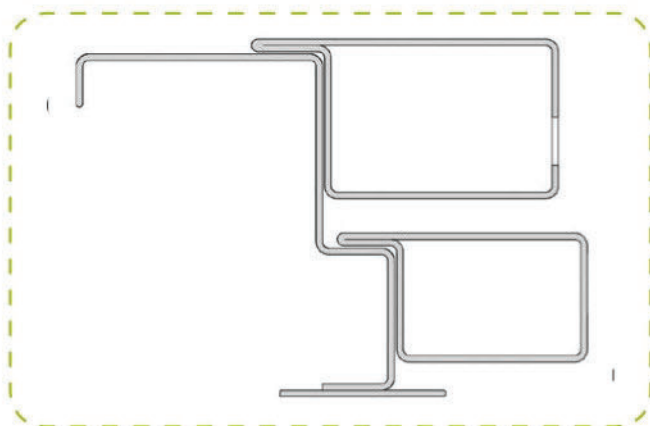
Dettaglio profilo scatolato telaio fisso ed anta
