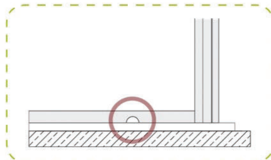
1. Sezione circolare per il deflusso dell'acqua piovana
